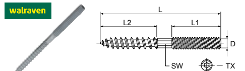
Srieginės smeigės su medisraigčiu, TORX, cinkuotos, WALRAVEN BIS hanger bolts, zinc, WALRAVEN
