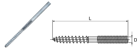
Srieginės smeigės SM, cinkuotos Hanger bolts SM, zinc
