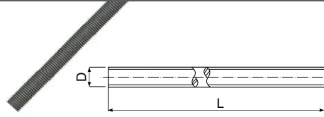
DIN975 – srieginiai strypai, karštai cinkuoti, 8.8 klasės DIN975 – threaded rods, hot-dip galvanized, 8.8 class
