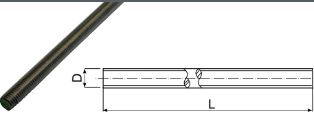
DIN975 – srieginiai strypai, juodi, 10.9 klasės DIN975 – threaded rods, without surface, 10.9 class
